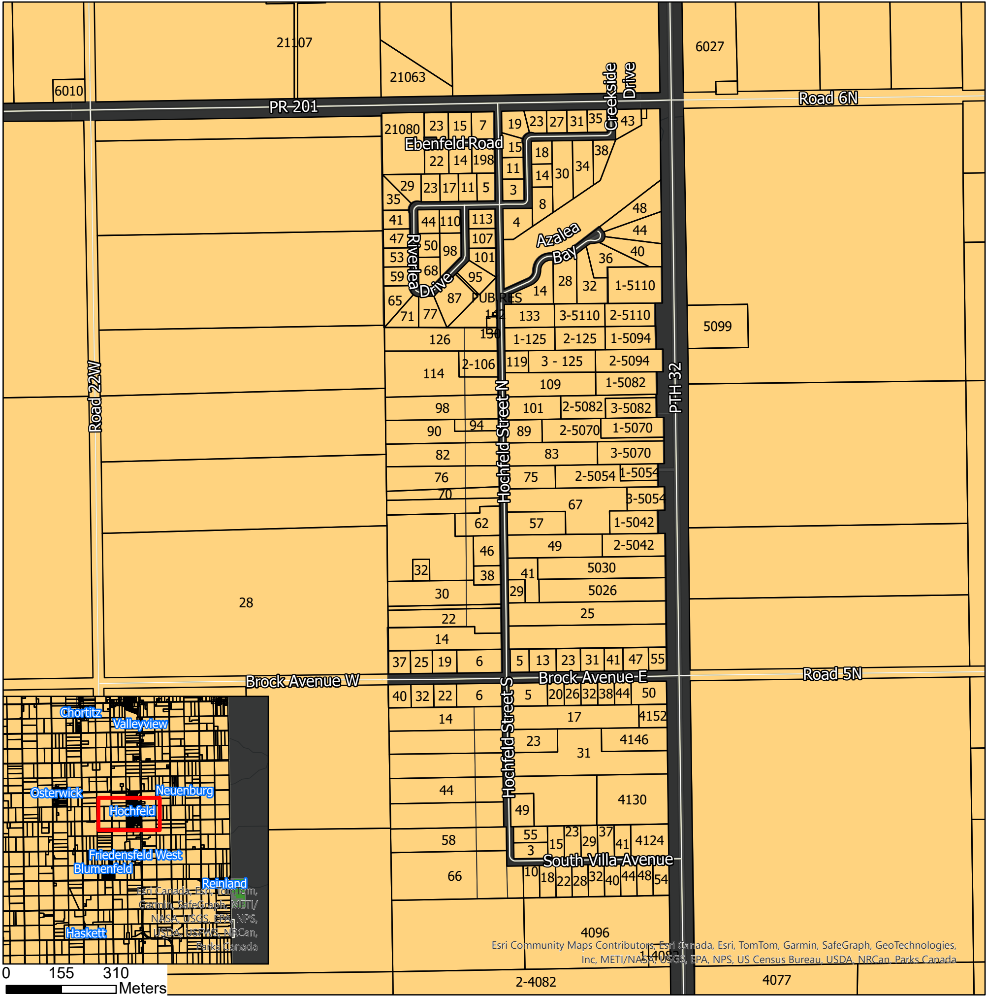
Hochfeld map
